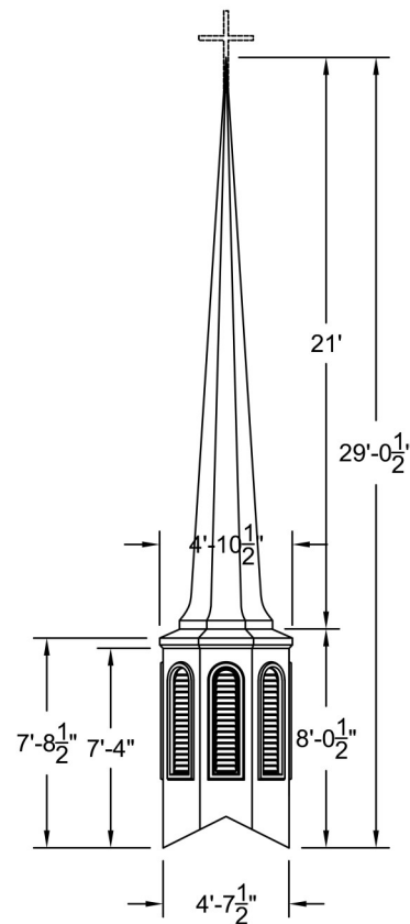
ELEVATION Scale: 5/32" = 1'-0"
