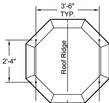
Plan View A-A Scale: 3/8" = 1'-0"
